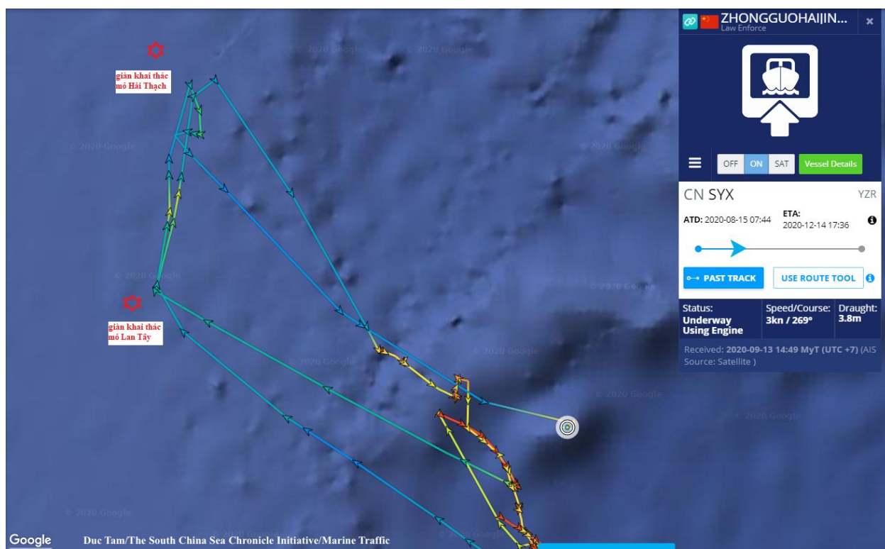
Sơ đồ hoạt động của Hải cảnh 5204 từ ngày 7 - 13/9/2020. Ảnh: Đức Tâm/Dự án Đại Sự Ký Biển Đông/Marine Traffic
