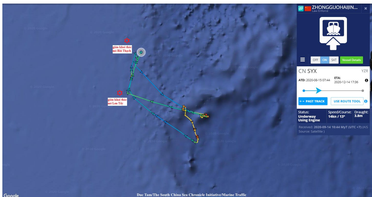
Sơ đồ hoạt động của Hải cảnh 5204 ngày 14/9/2020. Ảnh: Đức Tâm/Dự án Đại Sự Ký Biển Đông/Marine Traffic
