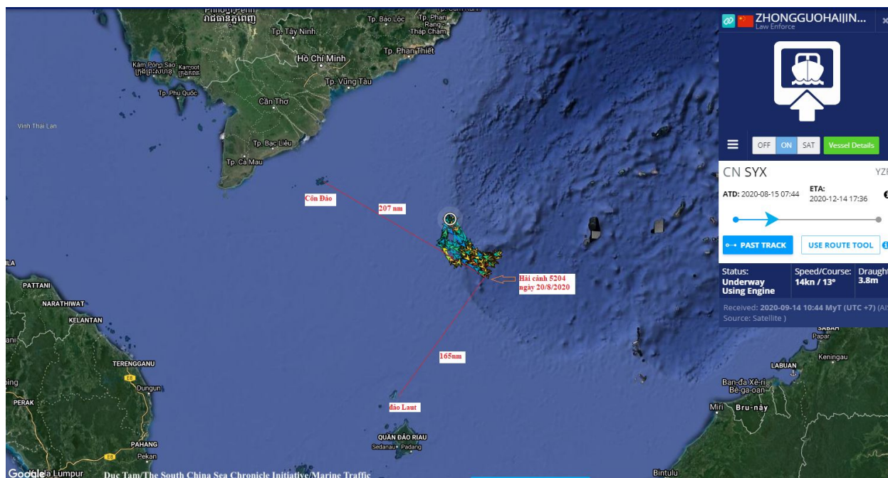
Khu vực hoạt động của Hải cảnh 5204 so với vùng biển Việt Nam và Indonesia. Ảnh: Đức Tâm/Dự án Đại Sự Ký Biển Đông/Marine Traffic
